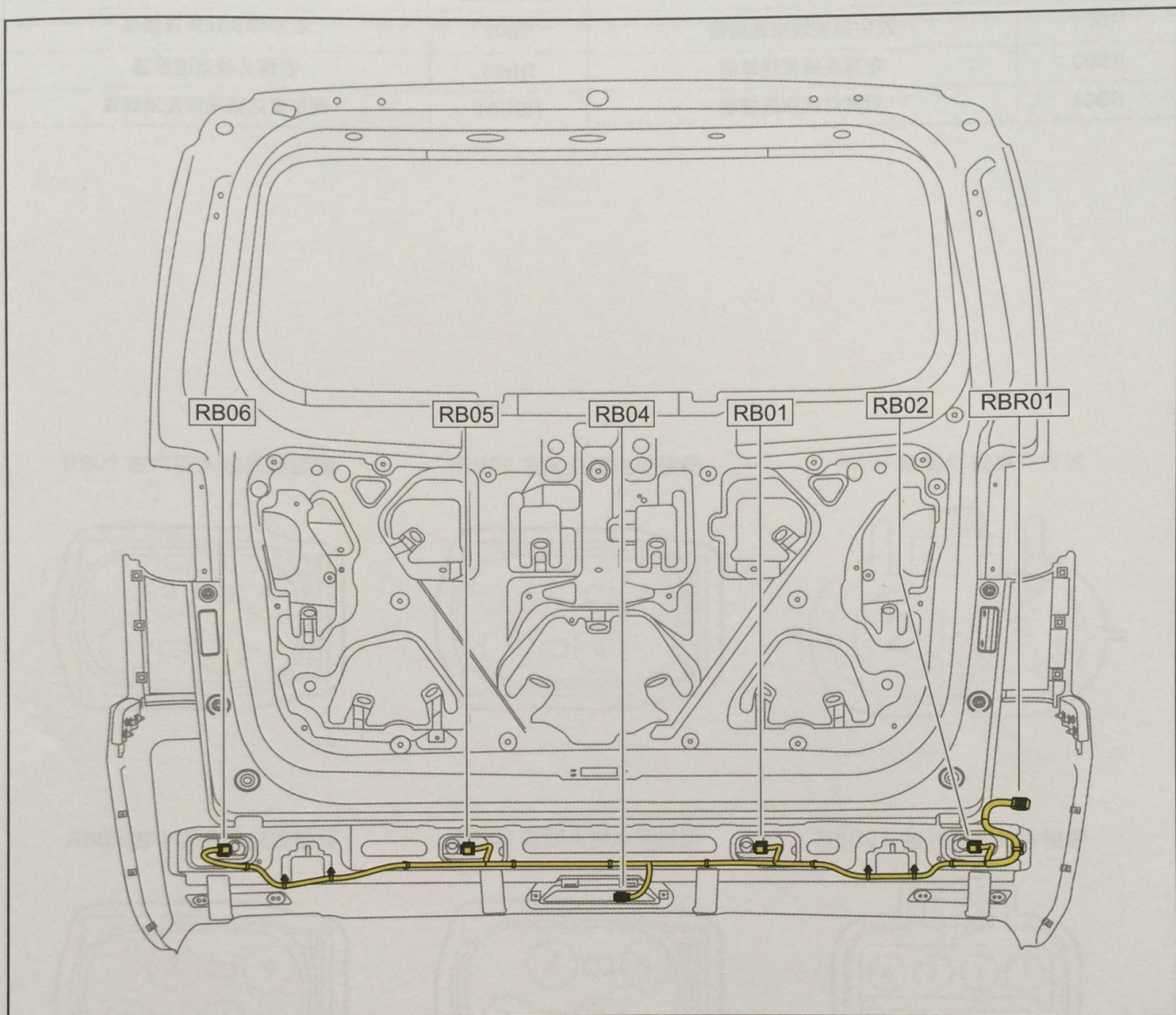
倒车雷达线束布置图
